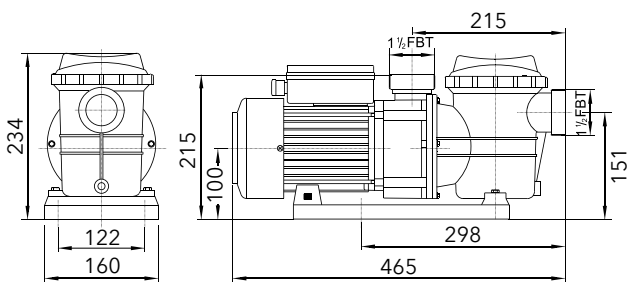
SMP - 10
